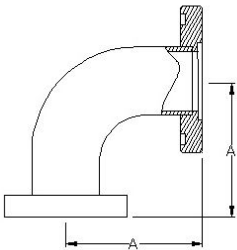
I013-ISO 90° ELBOW
