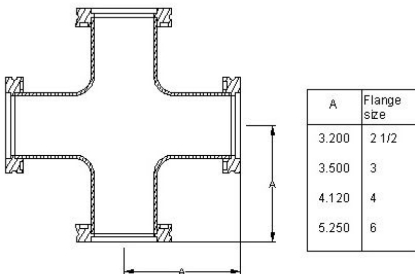
1019-ISO 4-way cross
